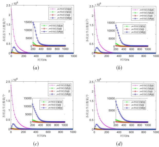
图5 不同免疫率 \omega 下Wiki-Talk网络中状态节点数量演化曲线:(a) \omega=0.82 (b) \omega=0.85 (c) \omega=0.88 (d) \omega=0.91
