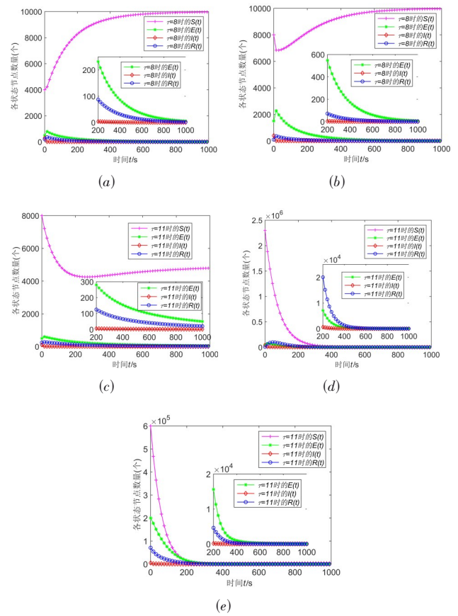
图3 R_0 < 1 时5个网络中状态节点数量随时间演化曲线:(a)ER 随机网络 (b)小世界网络 (c) P2P-Gnutella05 网络 (d) Wiki-Talk 网络 (e)Web-Google 网络
