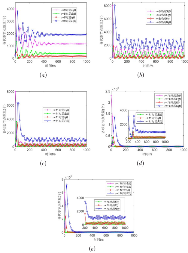
图2 R_0 > 1 时5个网络中状态节点数量随时间演化曲线:(a)ER 随机网络 (b)小世界网络 (c) P2P-Gnutella05 网络 (d) Wiki-Talk 网络 (e) Web-Google 网络
