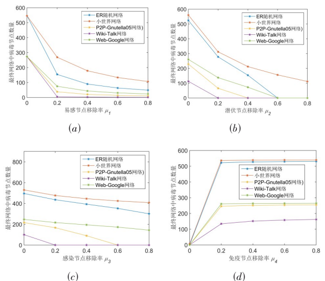
图6 节点移除率对病毒传播规模的影响:(a)易感节点移除率(b)潜伏节点移除率(c)感染节点移除率(d)免疫节点移除率
