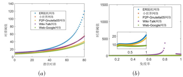
图4 不同参数对时滞阈值的影响:(a)潜伏时滞(b)免疫率
